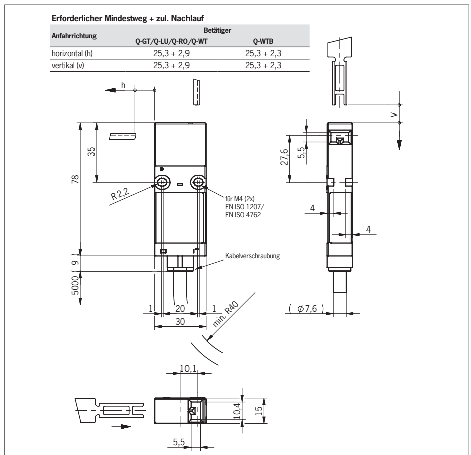
Bild 2: Maßzeichnung NQ..VZ
