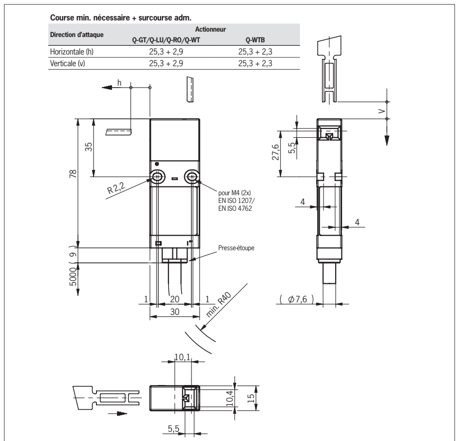
Fig. 2 : Dimensions NQ..VZ
