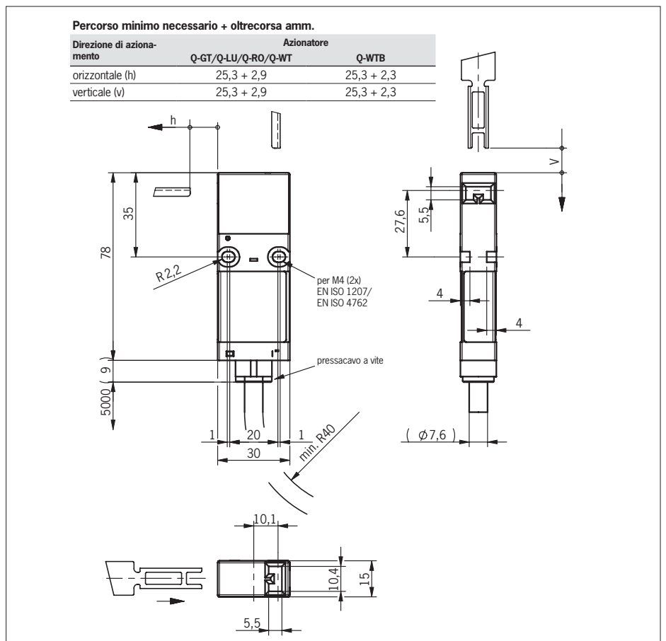
Fig. 2: Dimensioni NQ..VZ
